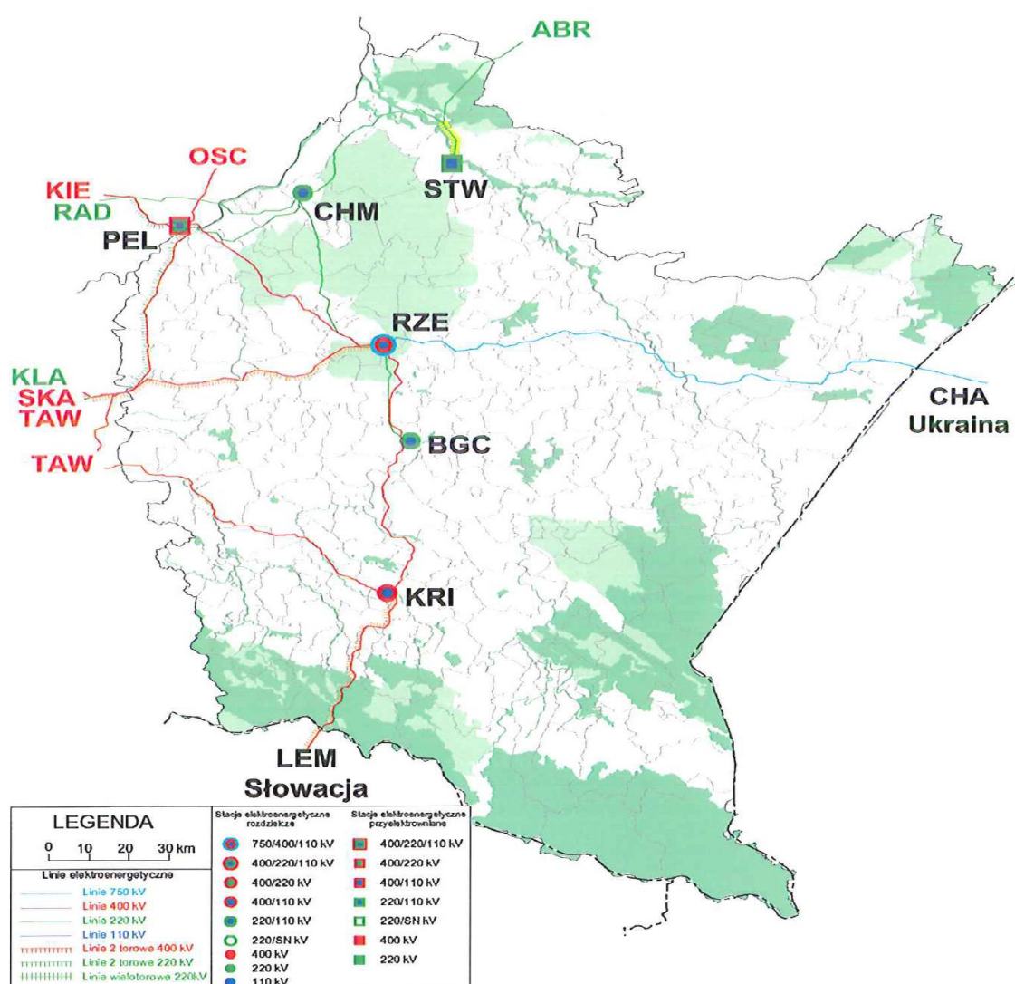
Rysunek 13 Schemat sieci przesyłowej z planami rozbudowy na rok 2025
