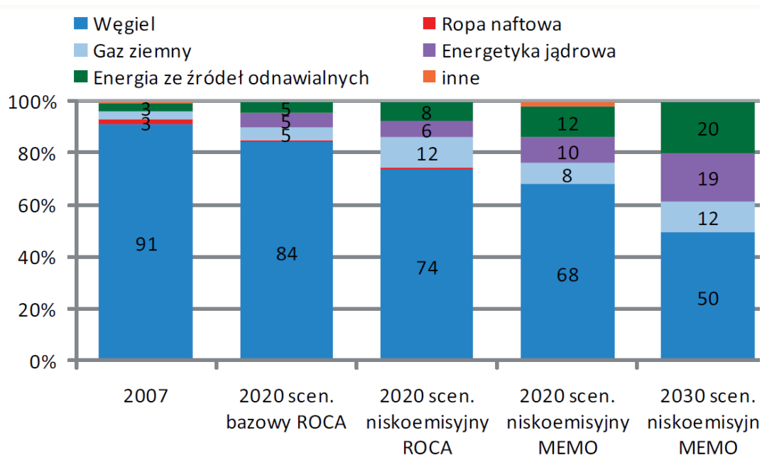
Rysunek 8 Obecna i prognozowana struktura źródeł wytwarzania energii elektrycznej w Polsce, w 2020 roku i 2030 roku
