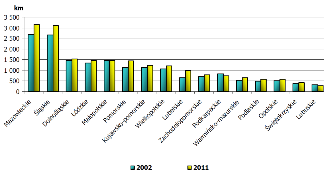
Rysunek 14 Długość sieci ciepłowniczej według województw
