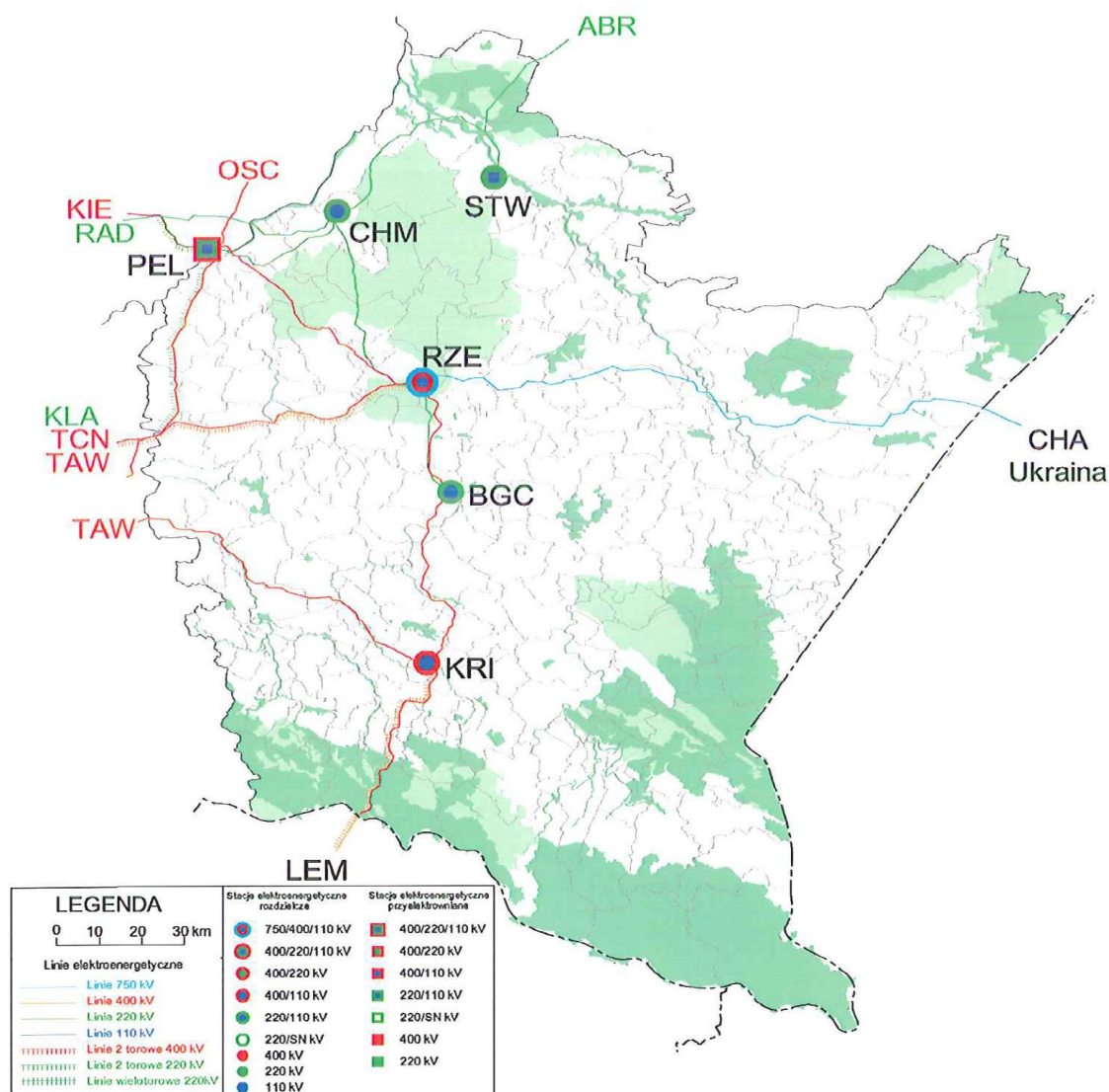
Rysunek 12 Schemat sieci przesyłowych stan na 2012 r.
