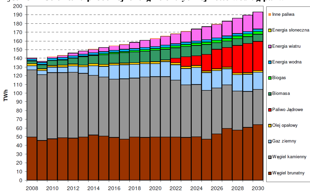
Rysunek 7 Struktura produkcji energii elektrycznej netto według paliw
