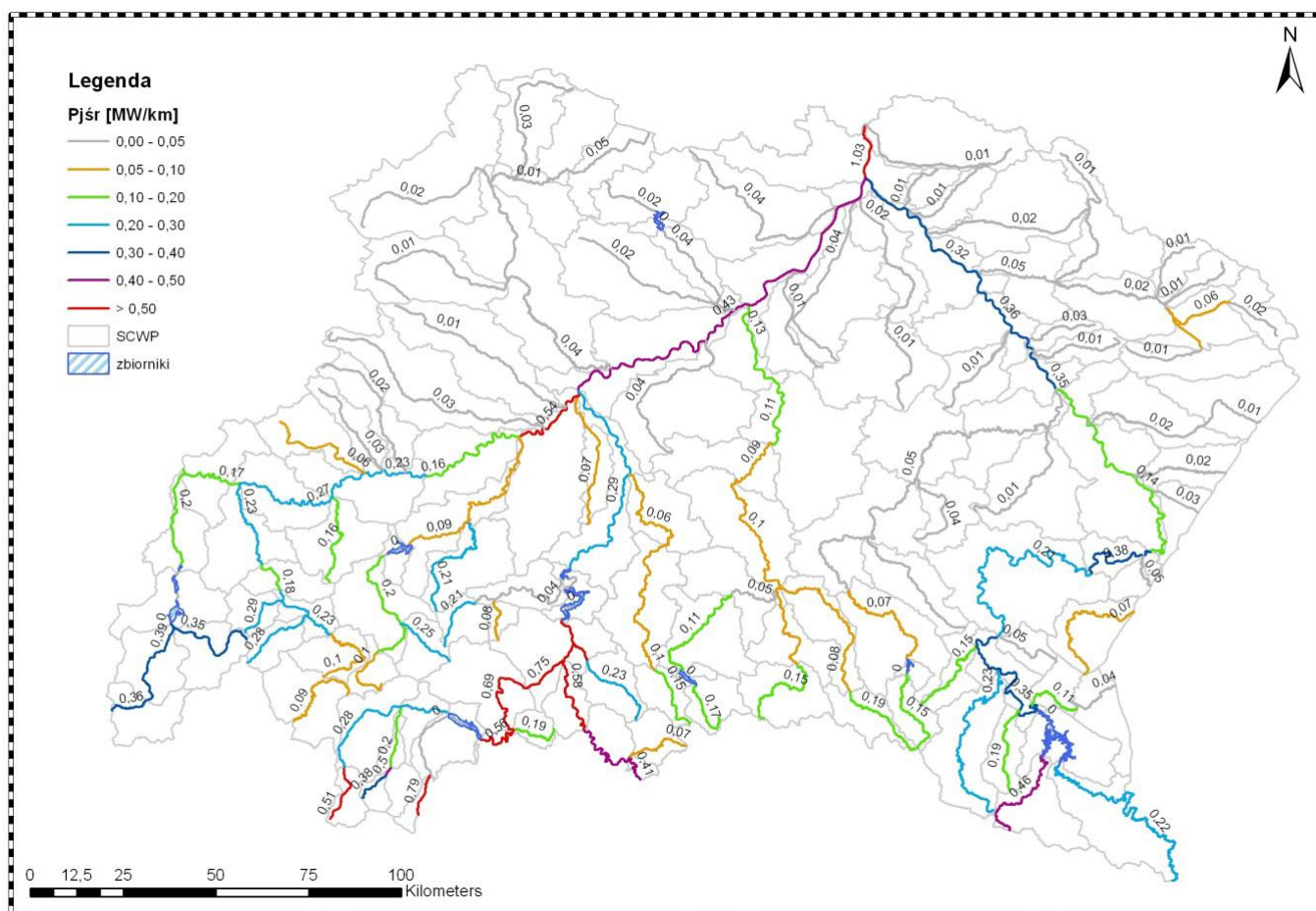
Rysunek 21 Potencjał teoretyczny głównych rzek będących w zarządzie RZGW Kraków
