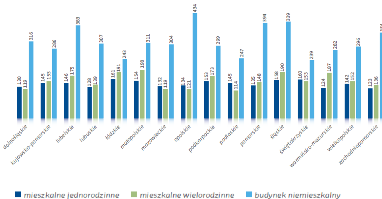
Rysunek 32. Zapotrzebowanie na energię pierwotną w budynkach w układzie wojewódzkim (kWh/m 2 /rok).
