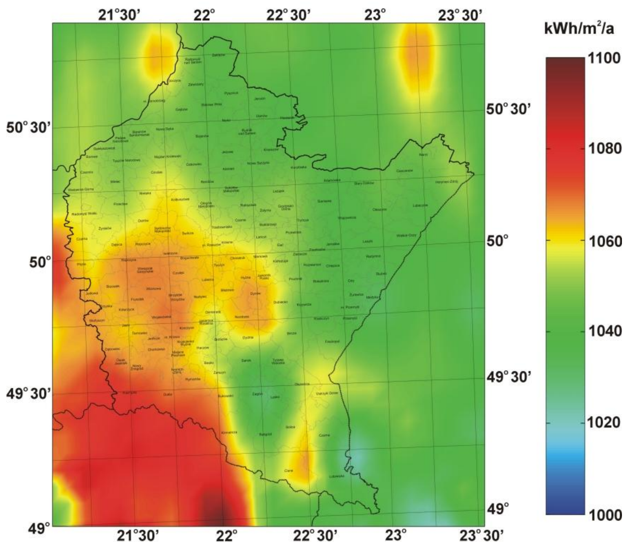
Rysunek 25. Rozkład przestrzenny całkowitego nasłonecznienia rocznego na terenie Podkarpacia.
