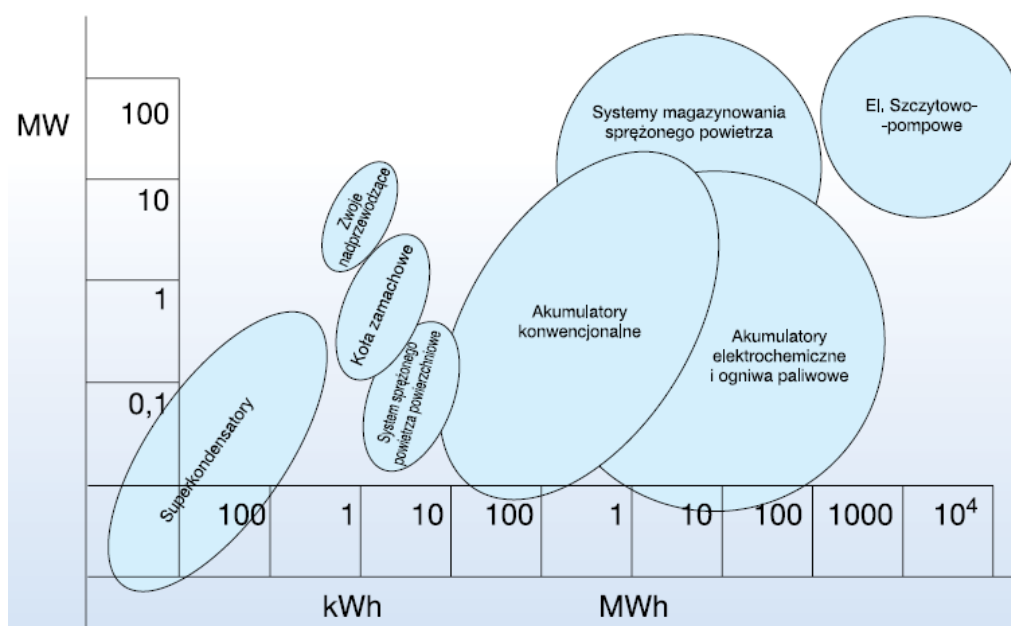
Rysunek 9 Rozkład typowych mocy jednostkowych i zdolności magazynowania dla wybranych grup technologii magazynowania energii
