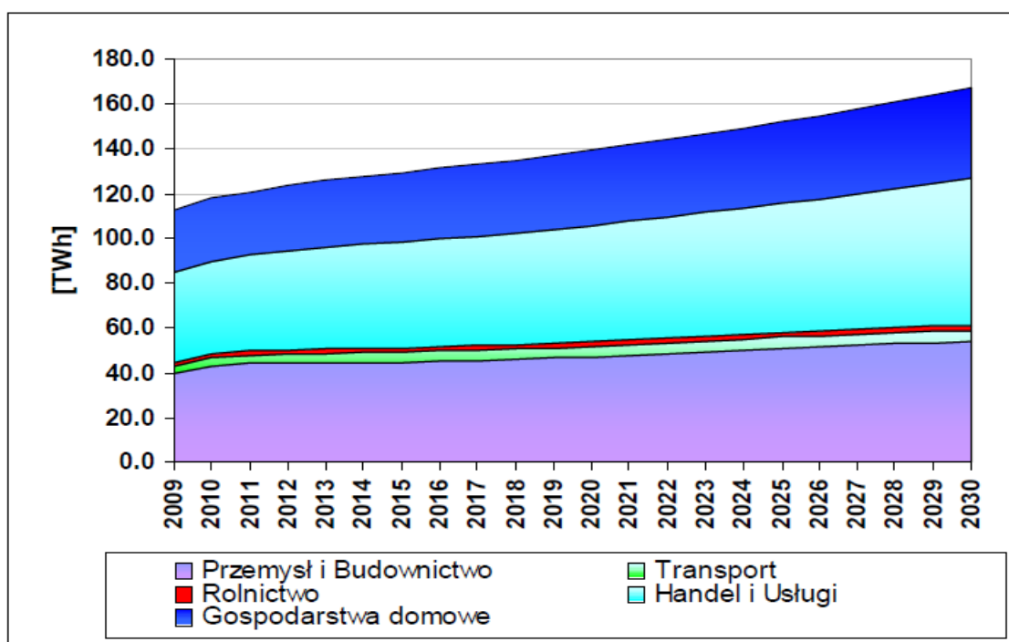
Rysunek 5 Prognoza zapotrzebowania finalnego na energię elektryczną w podziale na sektory
