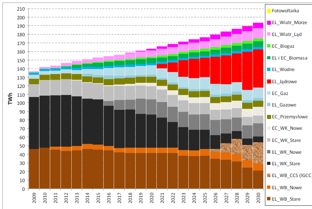
Rysunek 6 Prognozowana struktura produkcji energii elektrycznej netto
