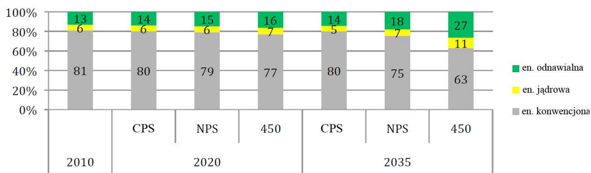
Rysunek 1 Udział źródeł energii według kategorii i scenariusz
