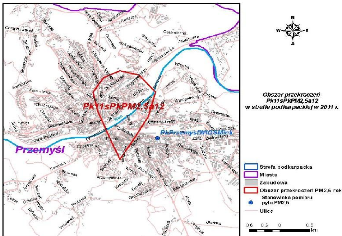
Rysunek 29. Obszar przekroczeń poziomu dopuszczalnego pyłu zawieszonego PM 2,5 rok Pk11sPkPM 2,5 a12 w strefie podkarpackiej w 2011 r.
