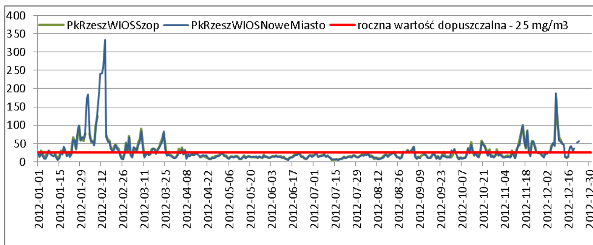
Rysunek 12 Roczny przebieg średnich dobowych wartości pyłu zawieszonego PM2,5 na stanowiskach pomiarowym w strefie miasto Rzeszów w 2012 r.
