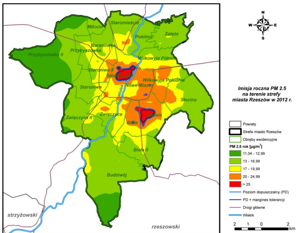
Stężenia PM2,5 o okresie uśredniania wyników rok w Rzeszowie pochodzące z łącznej emisji wszystkich typów w 2012 r.
