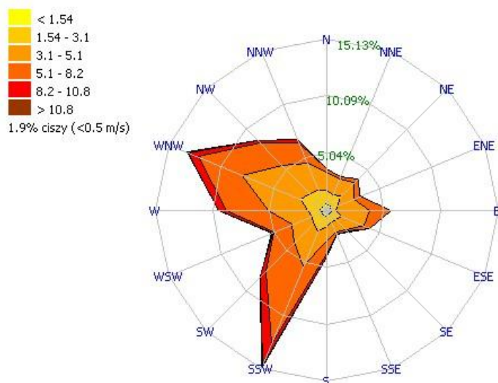
Rysunek 47 Rozkład kierunków i prędkości wiatru wyznaczony przez model WRF/CALMET w strefie miasto Rzeszów w 2012 r.
