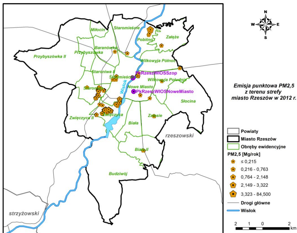
Rysunek 35 Emisja punktowa pyłu PM2,5 z terenu miasta Rzeszowa w 2012 r.
