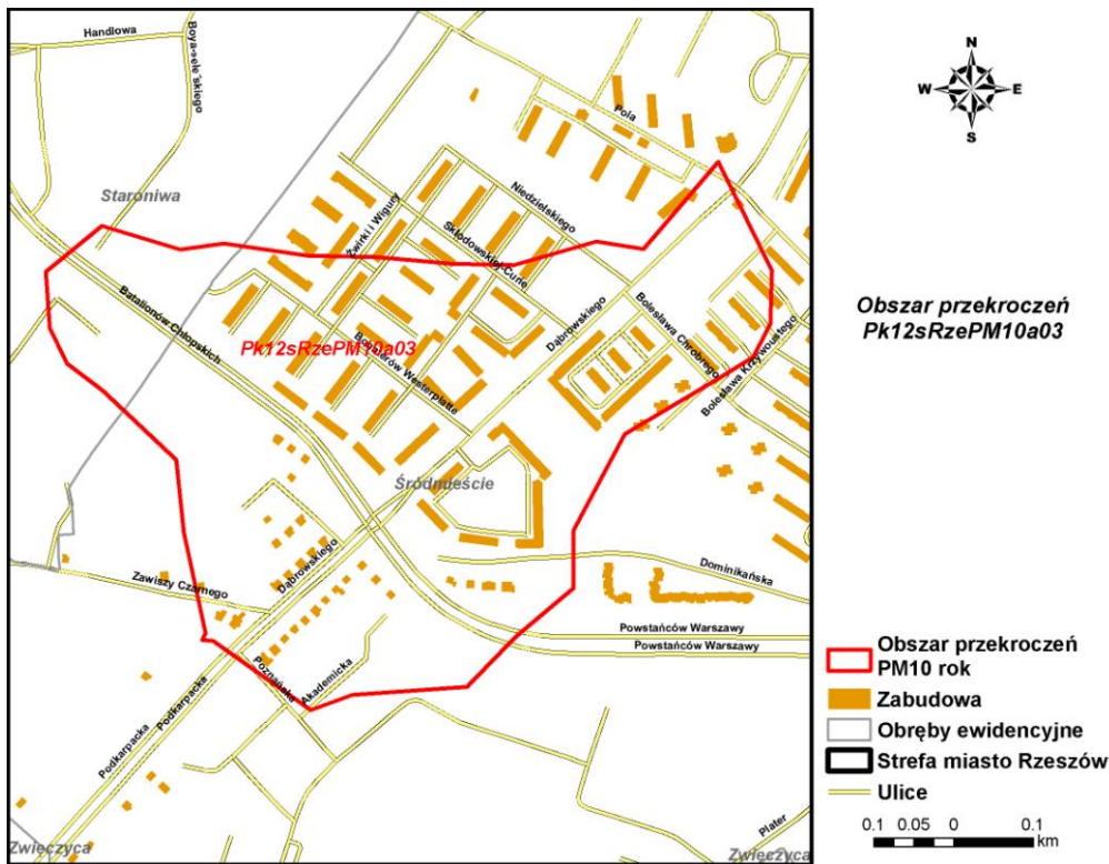
Rysunek 82 Obszar przekroczeń poziomu dopuszczalnego PM10 rok Pk12sRzePM10a03 w strefie miasto Rzeszów w 2012 r.
