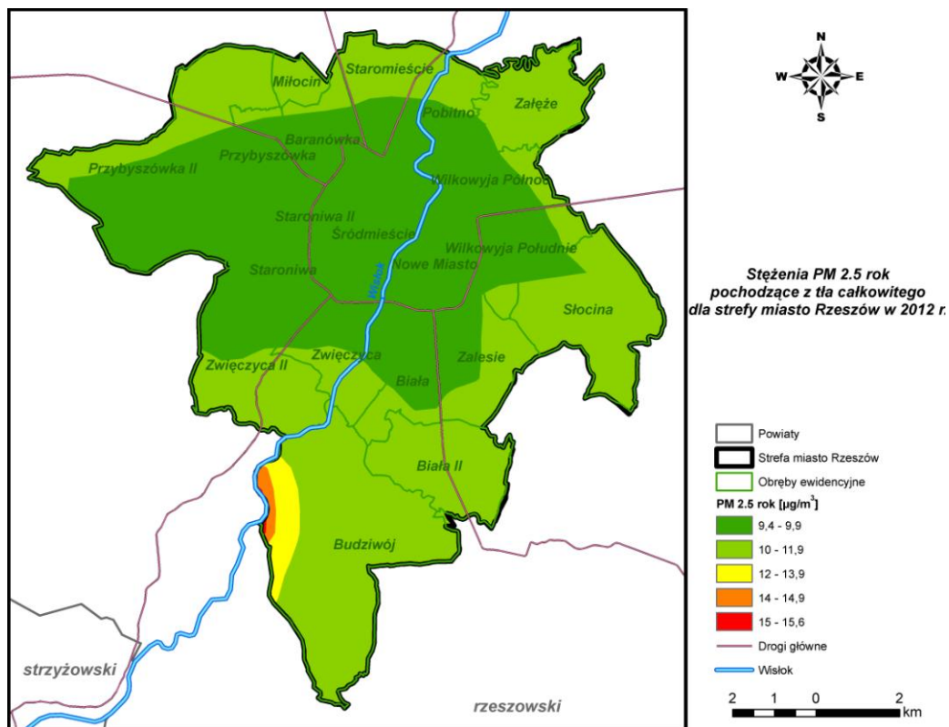
Rysunek 69 Stężenia pyłu PM2,5 o okresie uśredniania wyników rok w Rzeszowie pochodzące z tła całkowitego w 2012 r.
