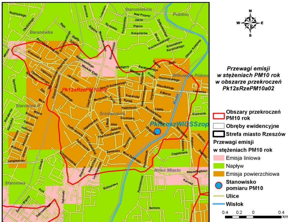
Rysunek 81 Przewagi typów emisji w stężeniach PM10 rok w obszarze przekroczeń Pk12sRzePM10a02 w strefie miasto Rzeszów w 2012 r.
