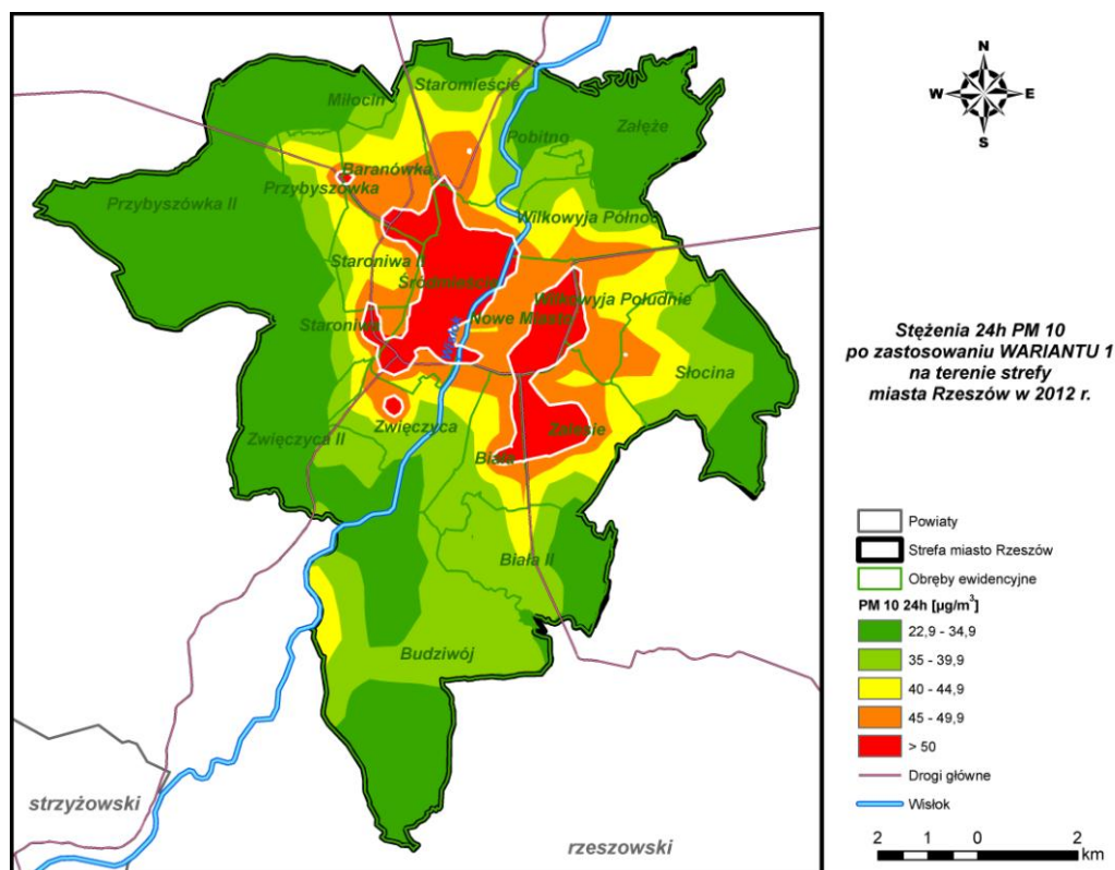
Rysunek 90 Stężenia PM10 o okresie uśredniania wyników 24 h w Rzeszowie pochodzące z łącznej emisji wszystkich typów po zastosowaniu założeń wariantu optymalnego
