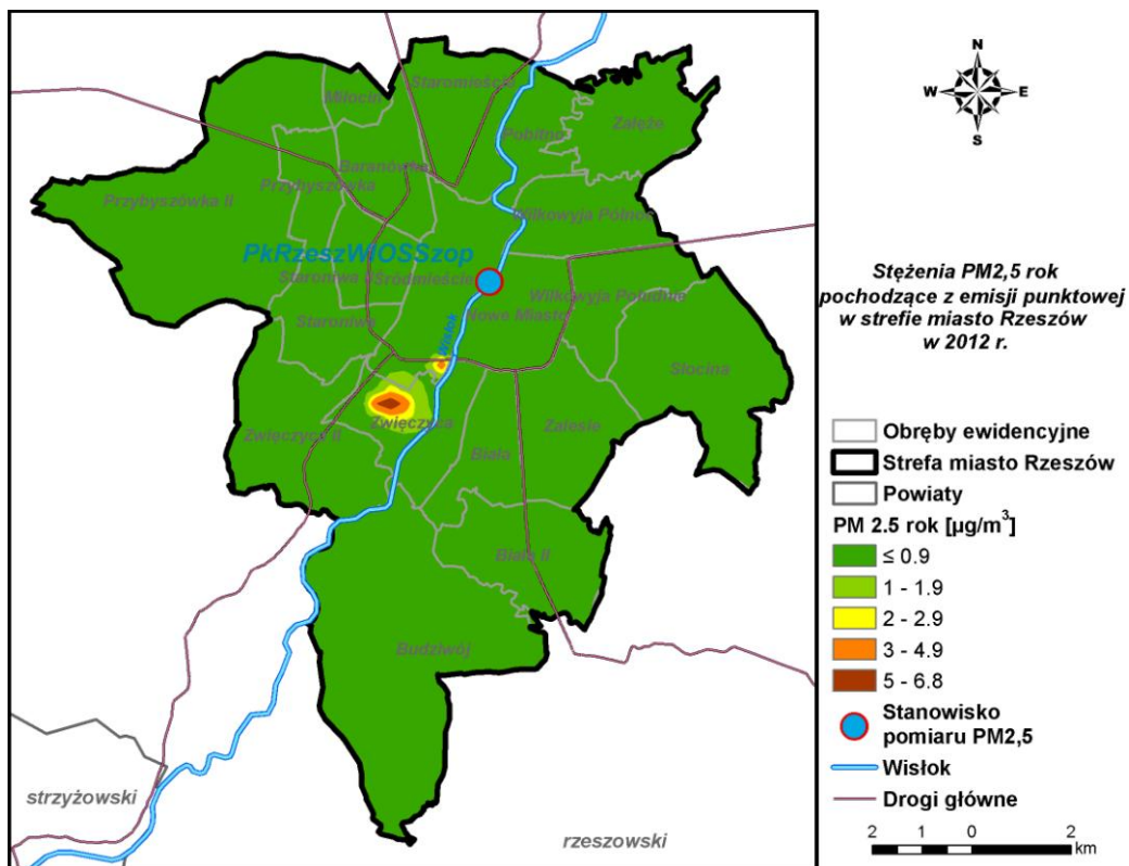
Rysunek 70 Stężenia pyłu zawieszonego PM 2,5 o okresie uśredniania wyników rok w Rzeszowie pochodzące z emisji punktowej w 2012 r.
