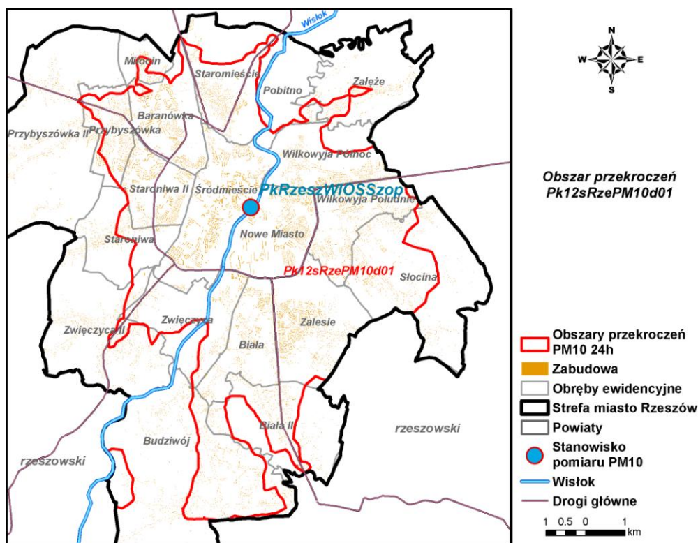
Rysunek 74 Obszar przekroczeń poziomu dopuszczalnego PM10 24h Pk12sRzePM10d01 w strefie miasto Rzeszów w 2012 r.
