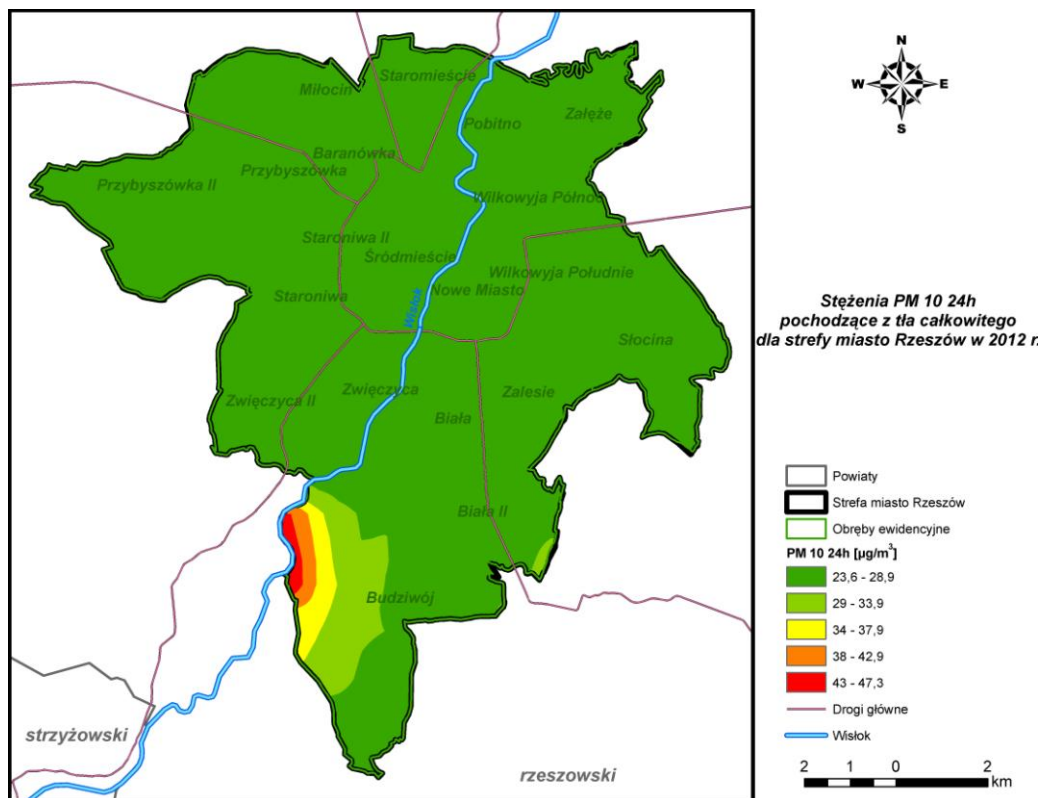
Rysunek 58 Stężenia pyłu PM10 o okresie uśredniania wyników 24h w Rzeszowie pochodzące z tła całkowitego w 2012 r.
