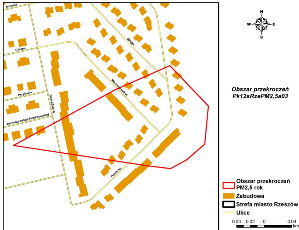
Rysunek 88 Obszar przekroczeń poziomu dopuszczalnego pyłu zawieszonego PM2,5 rok Pk12sRzePM2,5a03 w strefie miasto Rzeszów w 2012 r.
