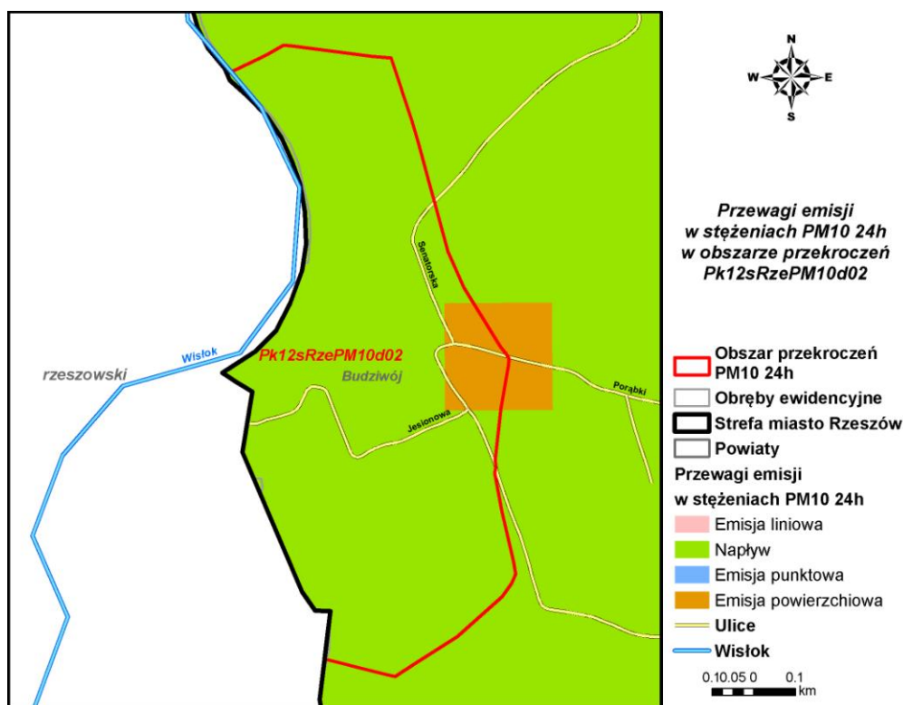
Rysunek 77 Przewagi typów emisji w stężeniach PM10 24h w obszarze przekroczeń Pk12sRzePM10d02 w strefie miasto Rzeszów w 2012 r.
