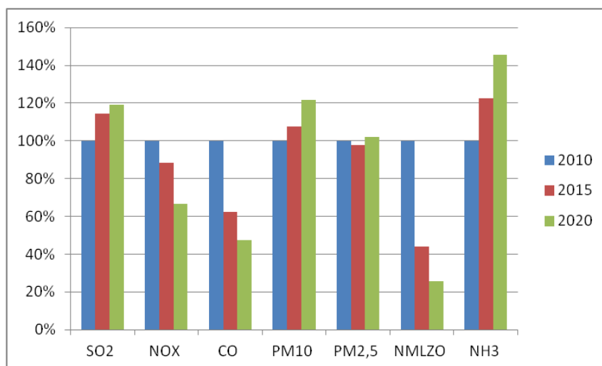
Rysunek 38 Prognoza emisji poszczególnych zanieczyszczeń pochodzących z komunikacji.
