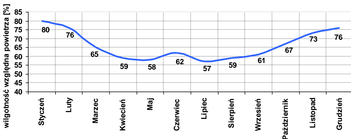
Rysunek 53 Średnia miesięczna wartość wilgotności względnej powietrza wyznaczona przez model WRF/CALMET w strefie miasto Rzeszów w 2012 r.
