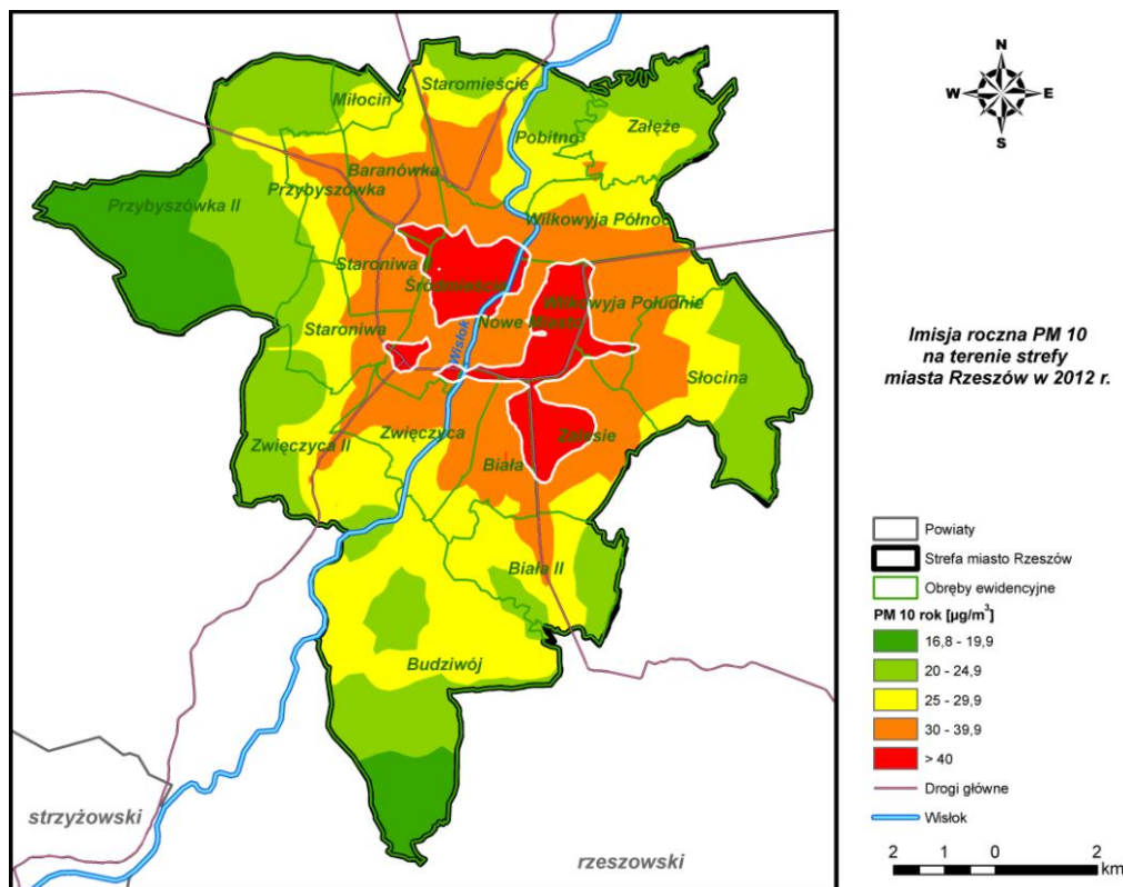
Rysunek 67 Stężenia pyłu zawieszonego PM10 o okresie uśredniania wyników rok w Rzeszowie pochodzące z łącznej emisji wszystkich typów w 2012 r.
