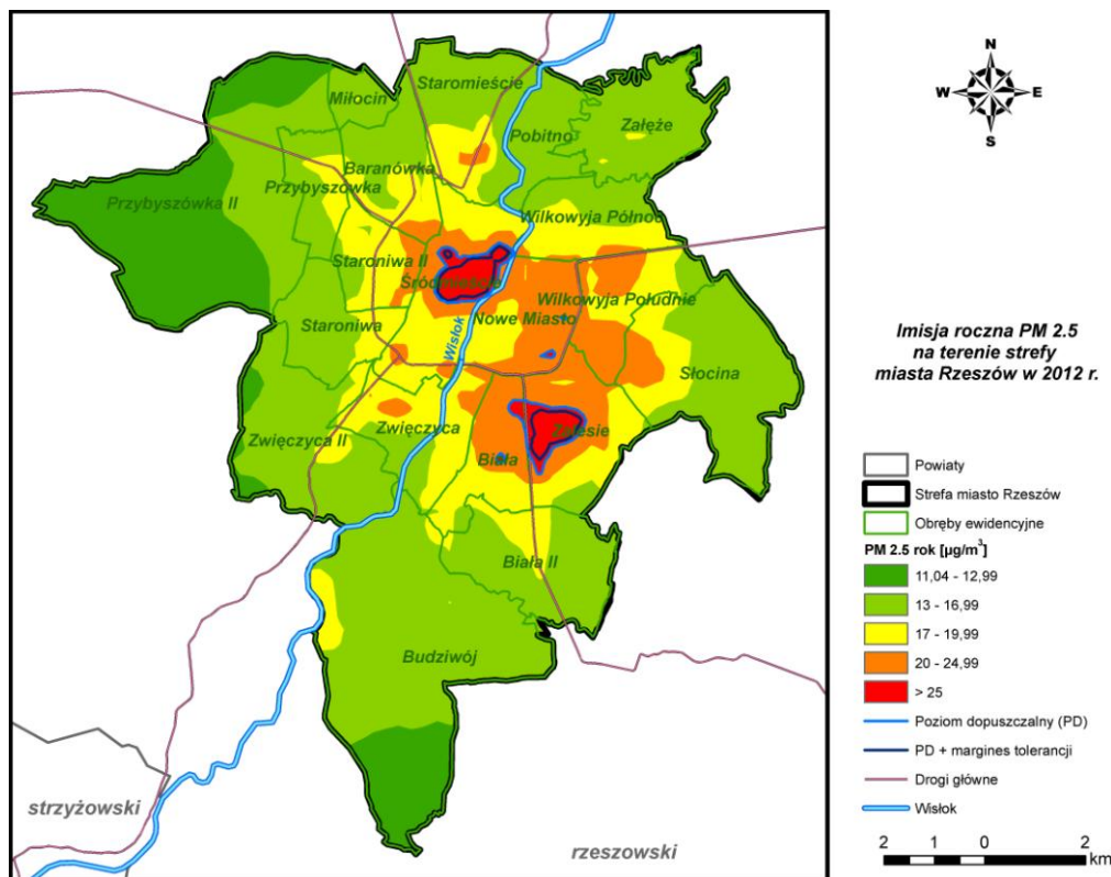
Rysunek 73 Stężenia pyłu zawieszonego PM 2,5 o okresie uśredniania wyników rok w Rzeszowie pochodzące z łącznej emisji wszystkich typów w 2012 r.
