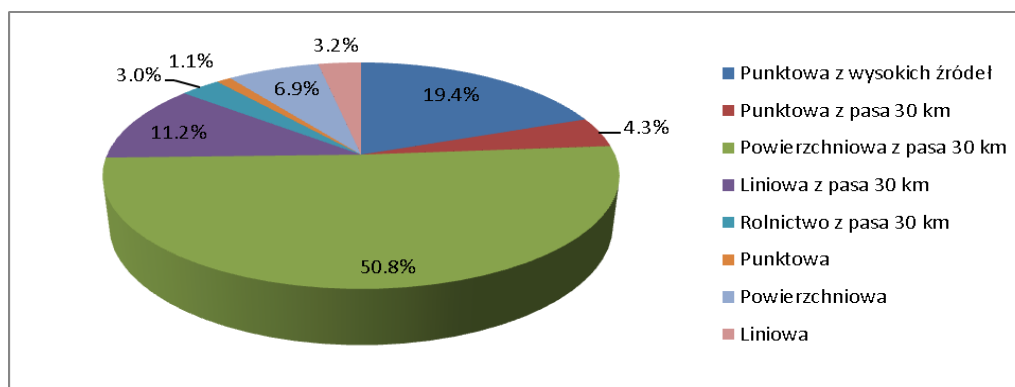
Rysunek 41 Procentowy udział typów źródeł w bilansie emisji pyłu PM10 dla strefy miasto Rzeszów w 2012 r.
