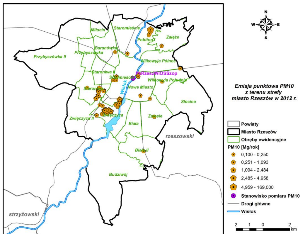
Rysunek 31 Emisja punktowa pyłu PM10 z terenu miasta Rzeszowa w 2012 r.
