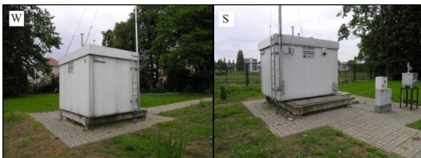
Rysunek 4 Otoczenie stanowiska pomiaru PM10 i PM 2,5 przy ul. Szopena w Rzeszowie
