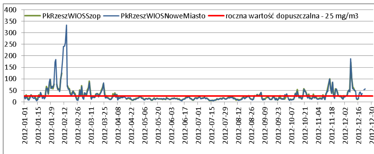
Roczny przebieg średnich dobowych wartości pyłu zawieszonego PM2,5 na stanowiskach pomiarowych w strefie miasto Rzeszów w 2012 r.
