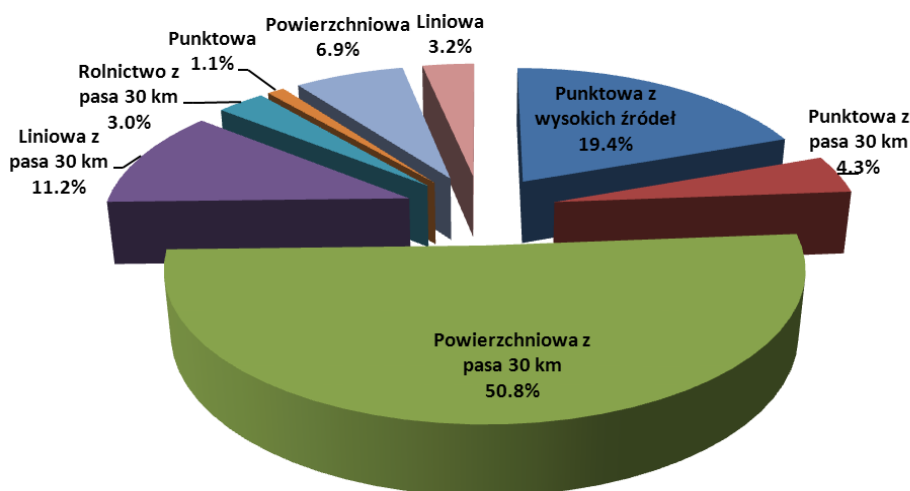
Procentowy udział typów źródeł w bilansie emisji PM10 dla strefy miasto Rzeszów w 2012 r.
