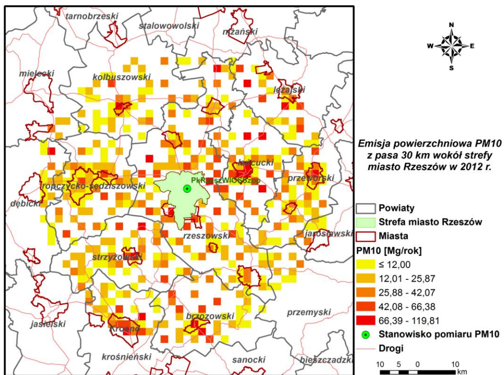
Rysunek 21 Emisja powierzchniowa pyłu PM10 z pasa 30 km wokół miasta Rzeszowa w 2012 r.
