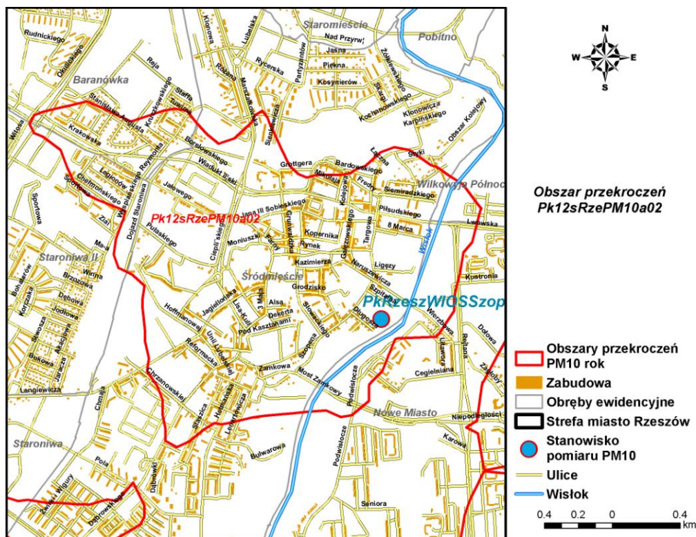
Rysunek 80 Obszar przekroczeń poziomu dopuszczalnego PM10 rok Pk12sRzePM10a02 w strefie miasto Rzeszów w 2012 r.
