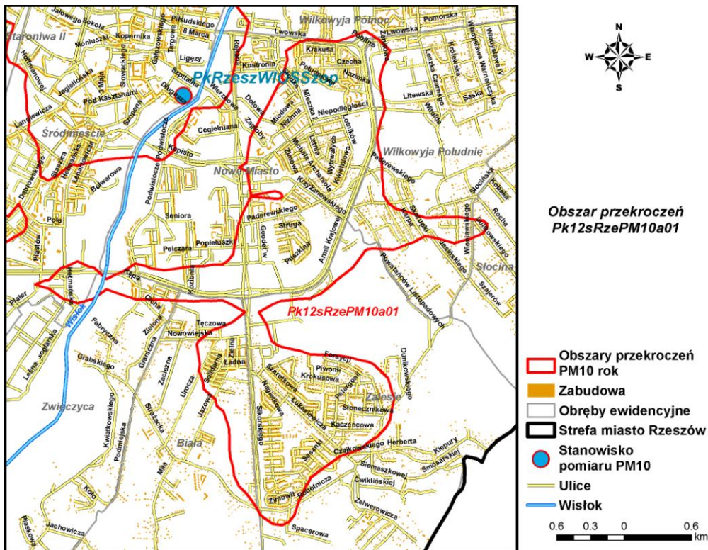
Rysunek 78 Obszar przekroczeń poziomu dopuszczalnego PM10 rok Pk12sRzePM10a01 w strefie miasto Rzeszów w 2012 r.
