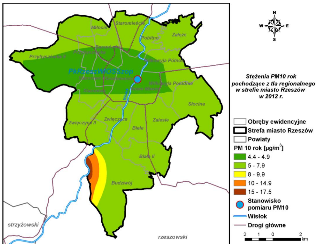
Rysunek 57 Stężenia pyłu zawieszonego PM10 o okresie uśredniania wyników rok w Rzeszowie pochodzące z tła regionalnego w 2012 r.
