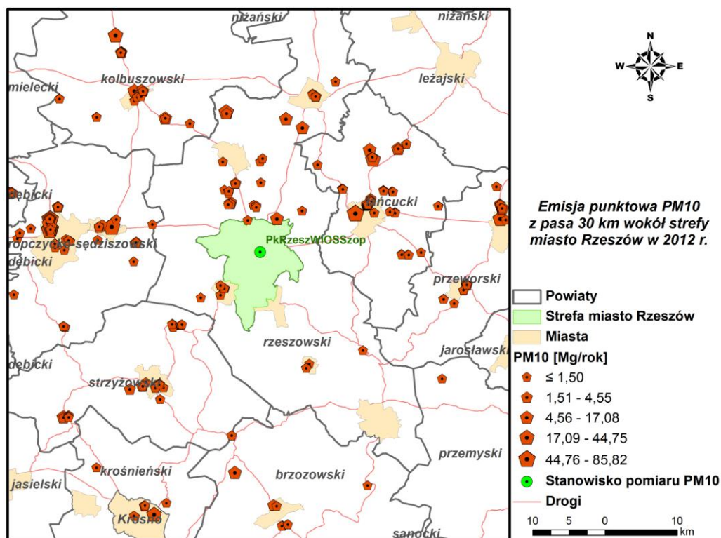
Rysunek 20 Emisja punktowa pyłu PM10 z pasa 30 km wokół miasta Rzeszowa w 2012 r.
