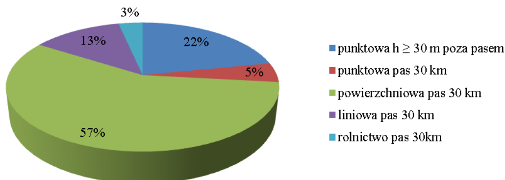
Rysunek 18 Udział procentowy poszczególnych typów emisji napływowej pyłu PM10 spoza strefy miast Rzeszów w 2012 r.
