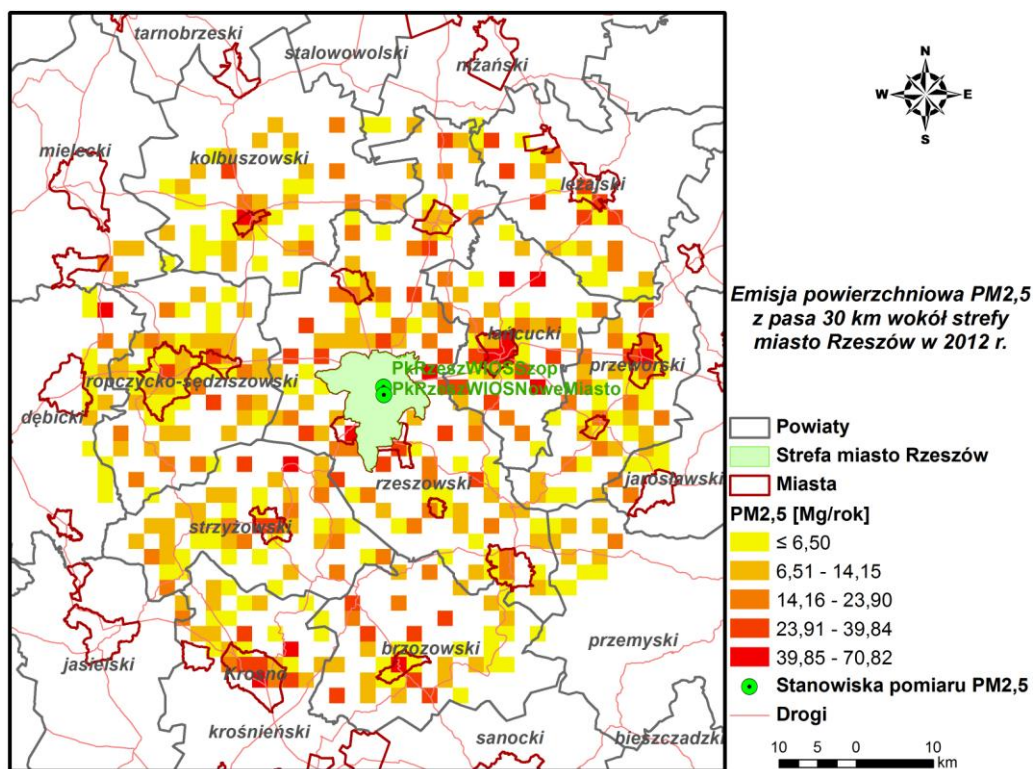
Rysunek 27 Emisja powierzchniowa pyłu PM2,5 z pasa 30 km wokół miasta Rzeszowa w 2012 r.
