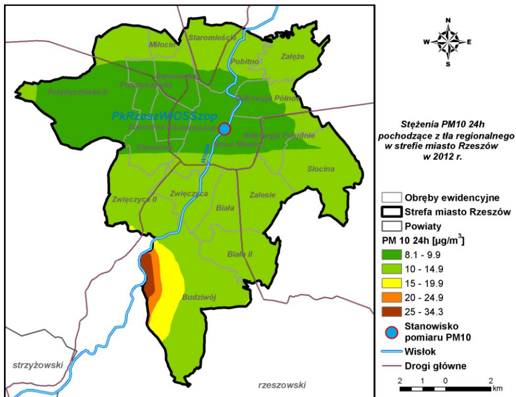
Rysunek 56 Stężenia PM10 o okresie uśredniania wyników 24h w strefie miasto Rzeszów pochodzące z tła regionalnego w 2012 r.
