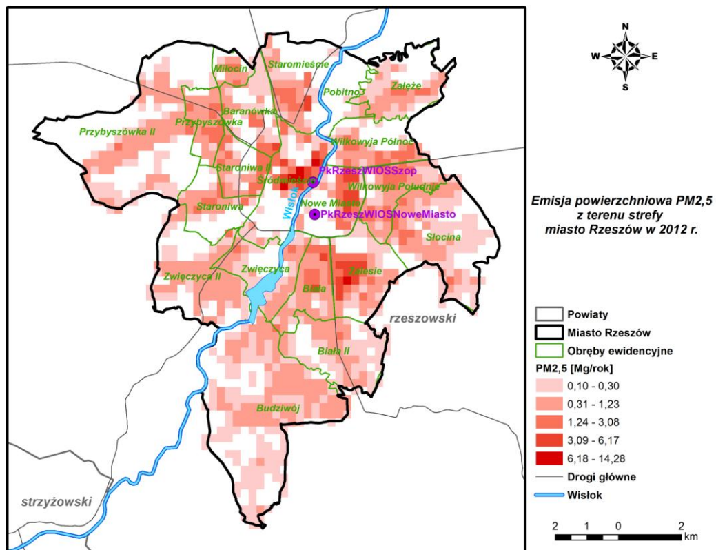
Rysunek 36 Emisja powierzchniowa pyłu PM 2,5 z terenu miasta Rzeszowa w 2012 r.
