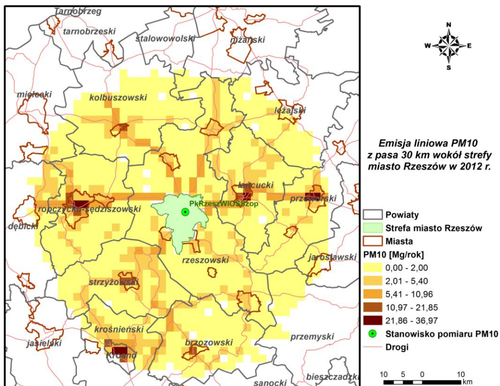
Rysunek 22 Emisja komunikacyjna pyłu PM10 z pasa 30 km wokół miasta Rzeszowa w 2012 r
