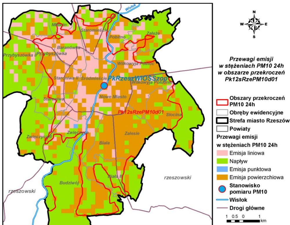
Rysunek 75 Przewagi typów emisji w stężeniach PM10 24h w obszarze przekroczeń Pk12sRzePM10d01 w strefie miasto Rzeszów w 2012 r.
