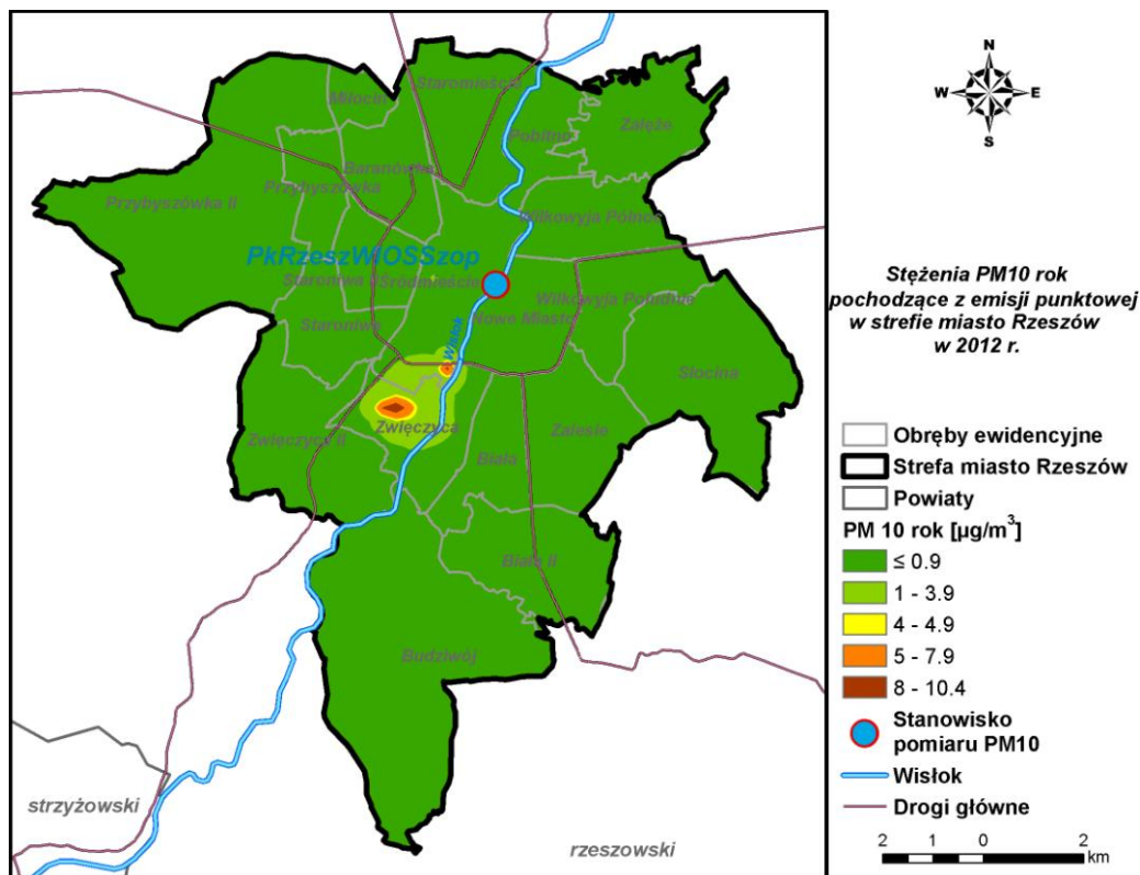
Rysunek 61 Stężenia pyłu zawieszonego PM10 o okresie uśredniania wyników rok w Rzeszowie pochodzące z emisji punktowej w 2012 r.
